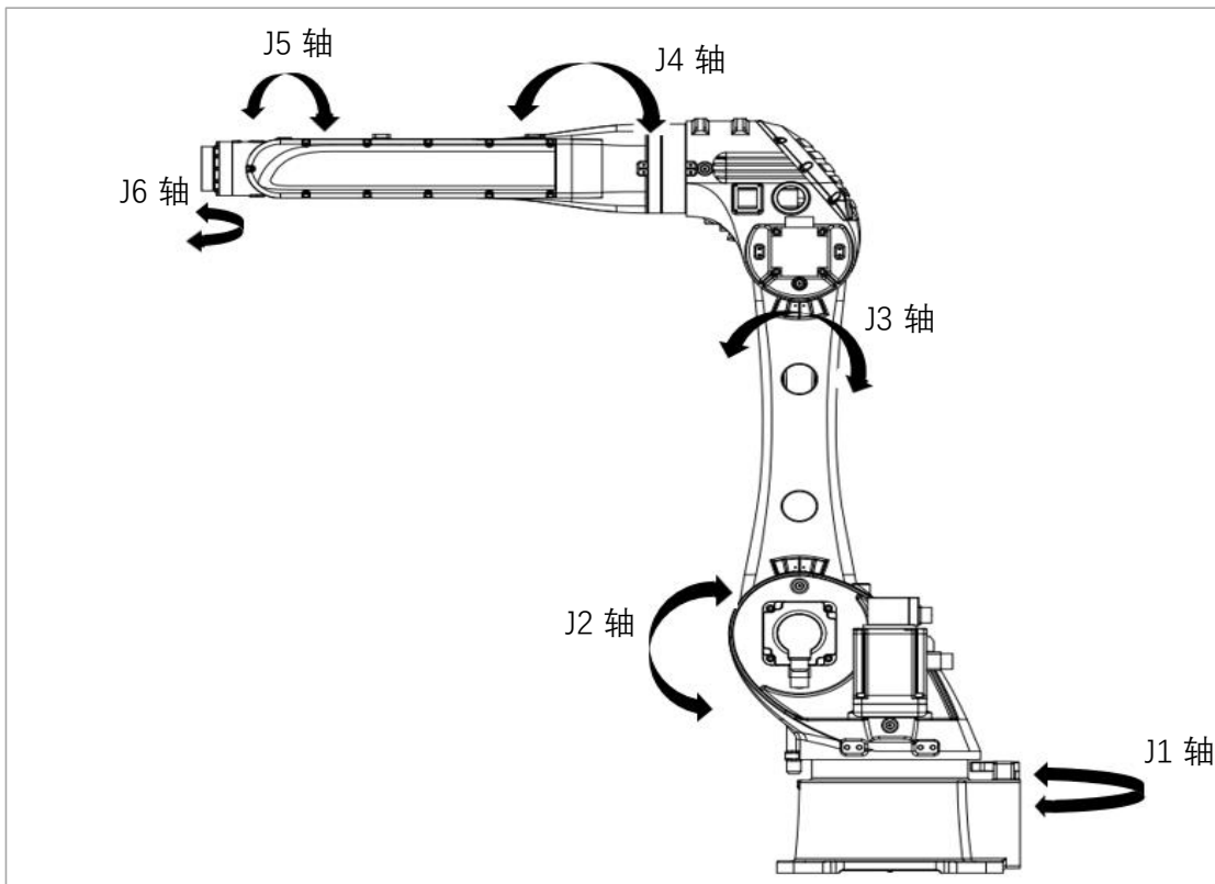
● MB38-1870 机器人动作方位示意图
