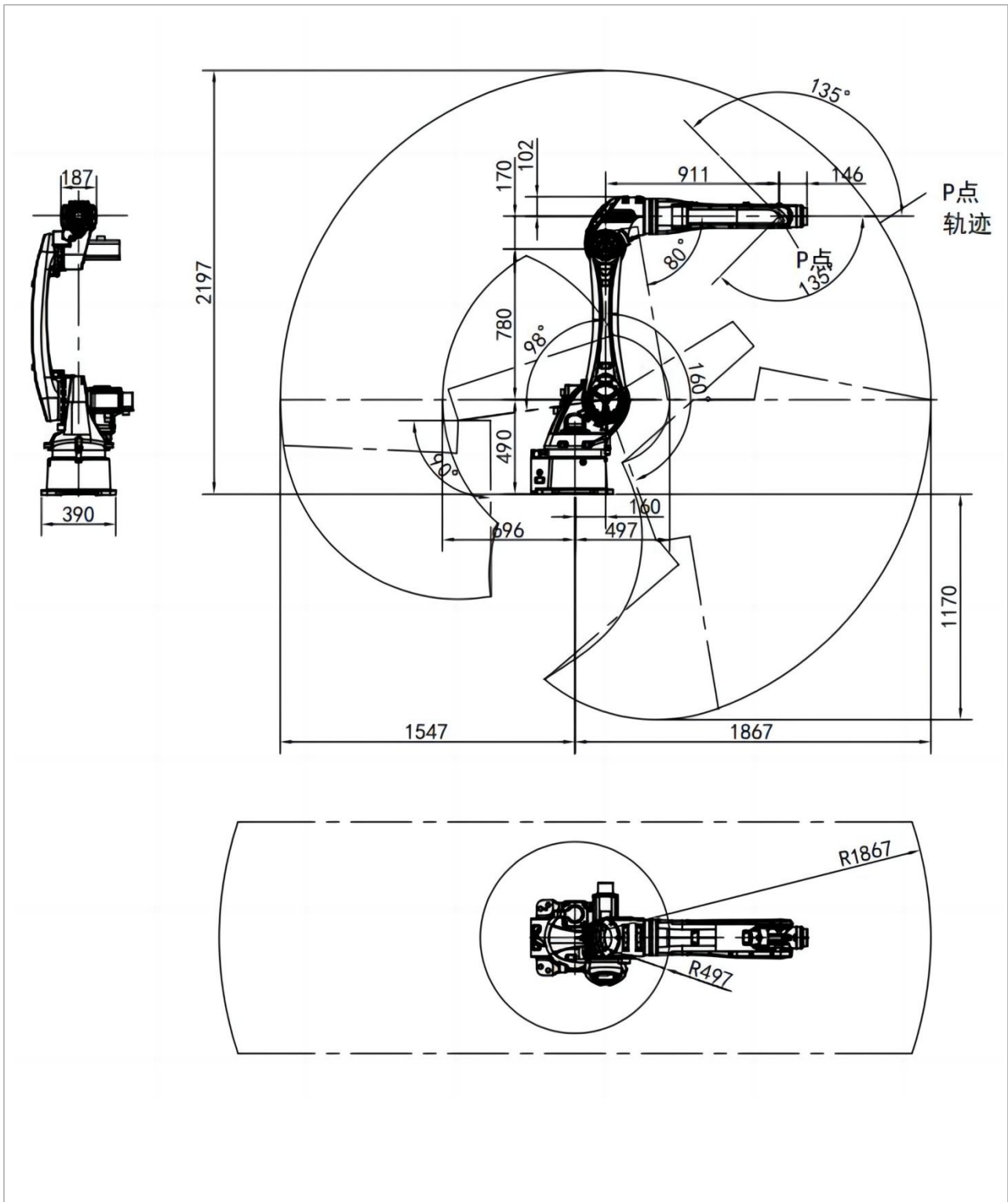
● MB38-1870 机器人外形尺寸及动作范围 (单位:mm 曲线部分:p 点动作范围)
