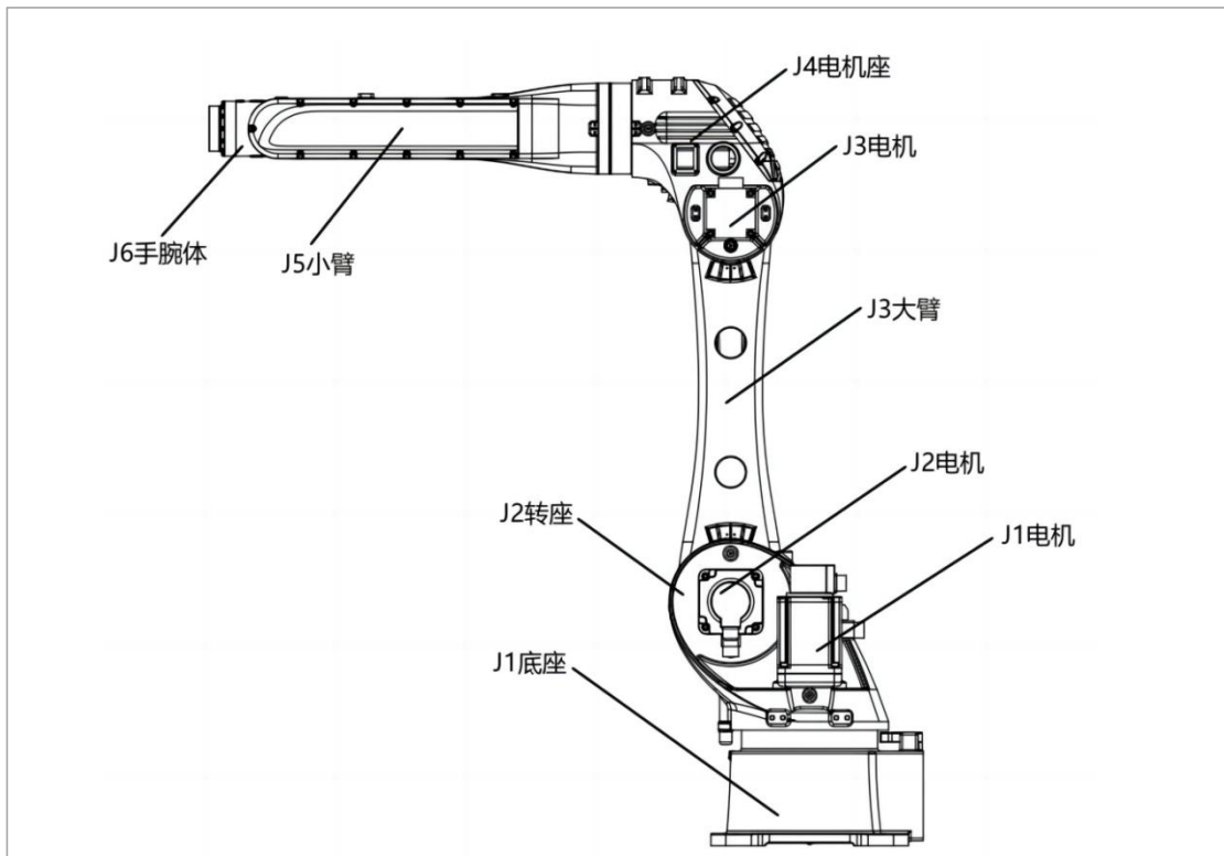
● MB38-1870 机器人构成图解
