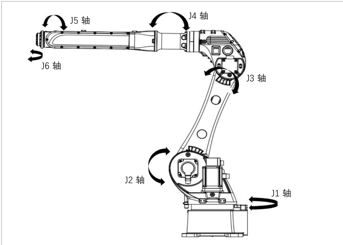
● MB20-2100 机器人动作方位示意图
