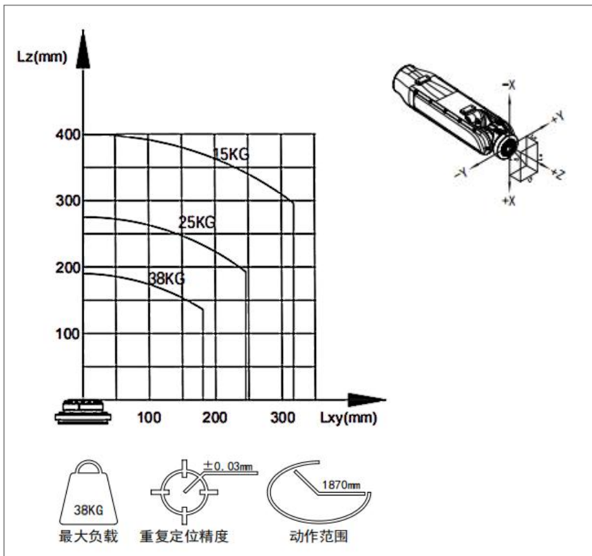
● MB38-1870 机器人腕部负载图
