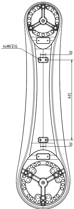
J3大臂安装尺寸 ◀
