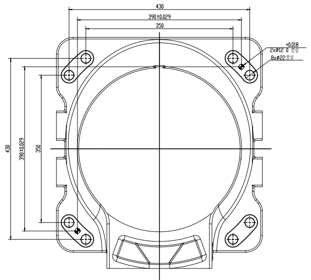
底座安装尺寸
