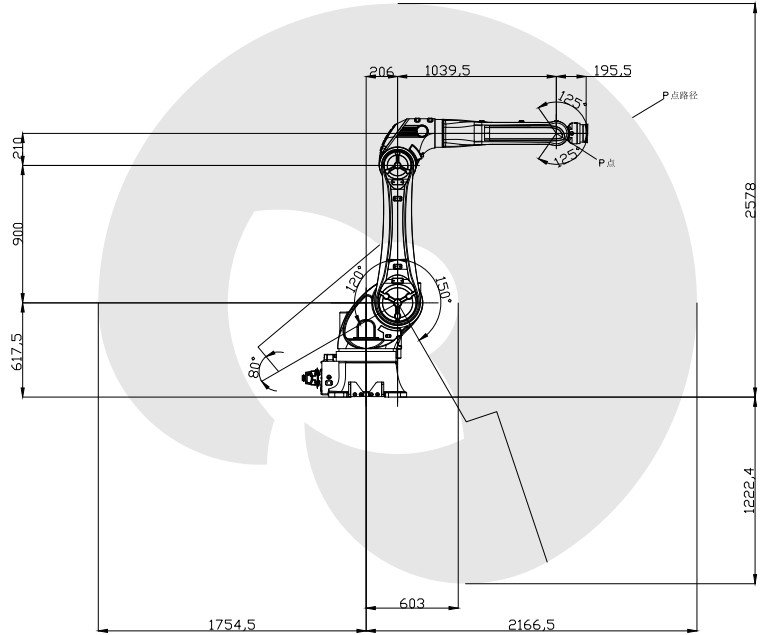
P点运动范围
