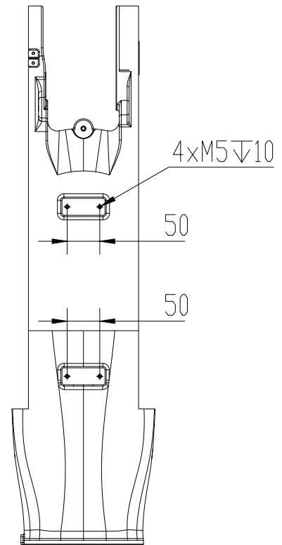
J5手腕体安装尺寸 ◀
