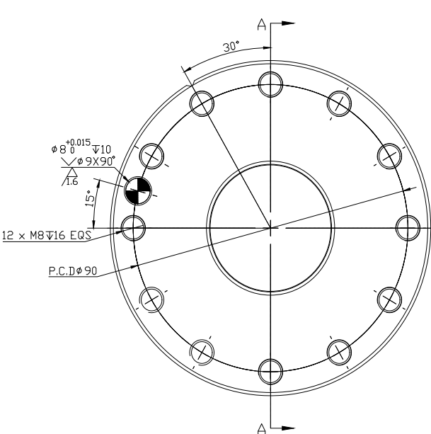
末端法兰安装尺寸
