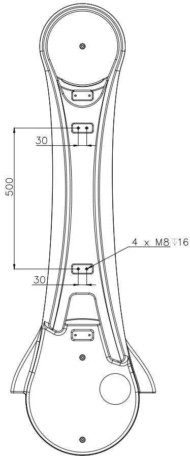
J3大臂安装尺寸 ◀
