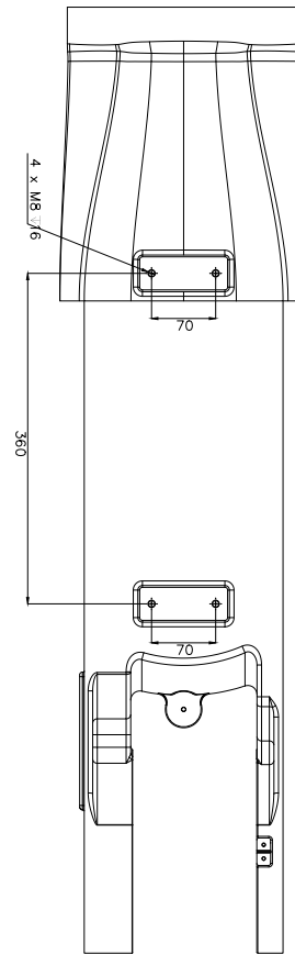
J5手腕体安装尺寸 ◀
