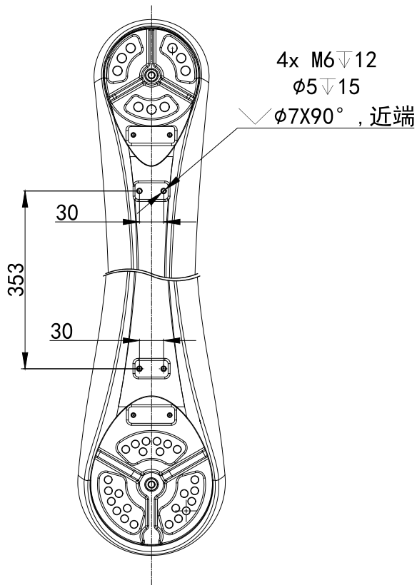
J3大臂安装尺寸
