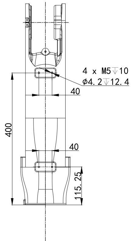
J5手腕体安装尺寸
