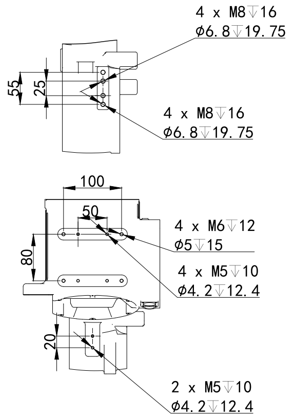
J4电机座安装尺寸
