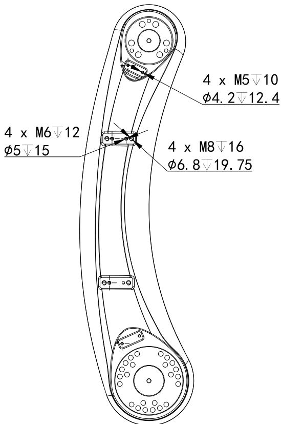
J3大臂安装尺寸
