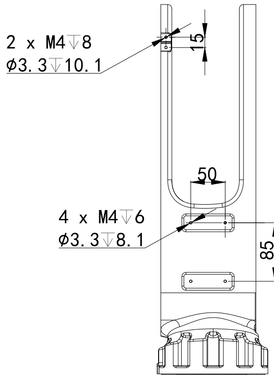
J5手腕体安装尺寸
